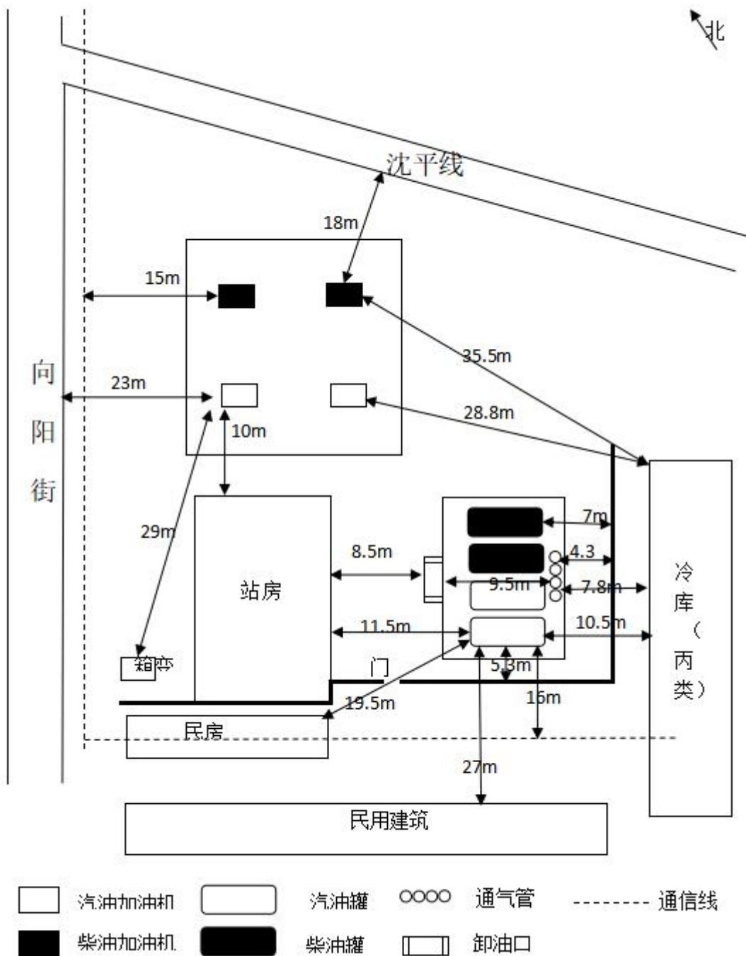
图 2.3-1 周边环境及总平面布置图
