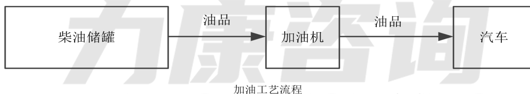
图 2.6-2 柴油卸油、加油工艺流程图
