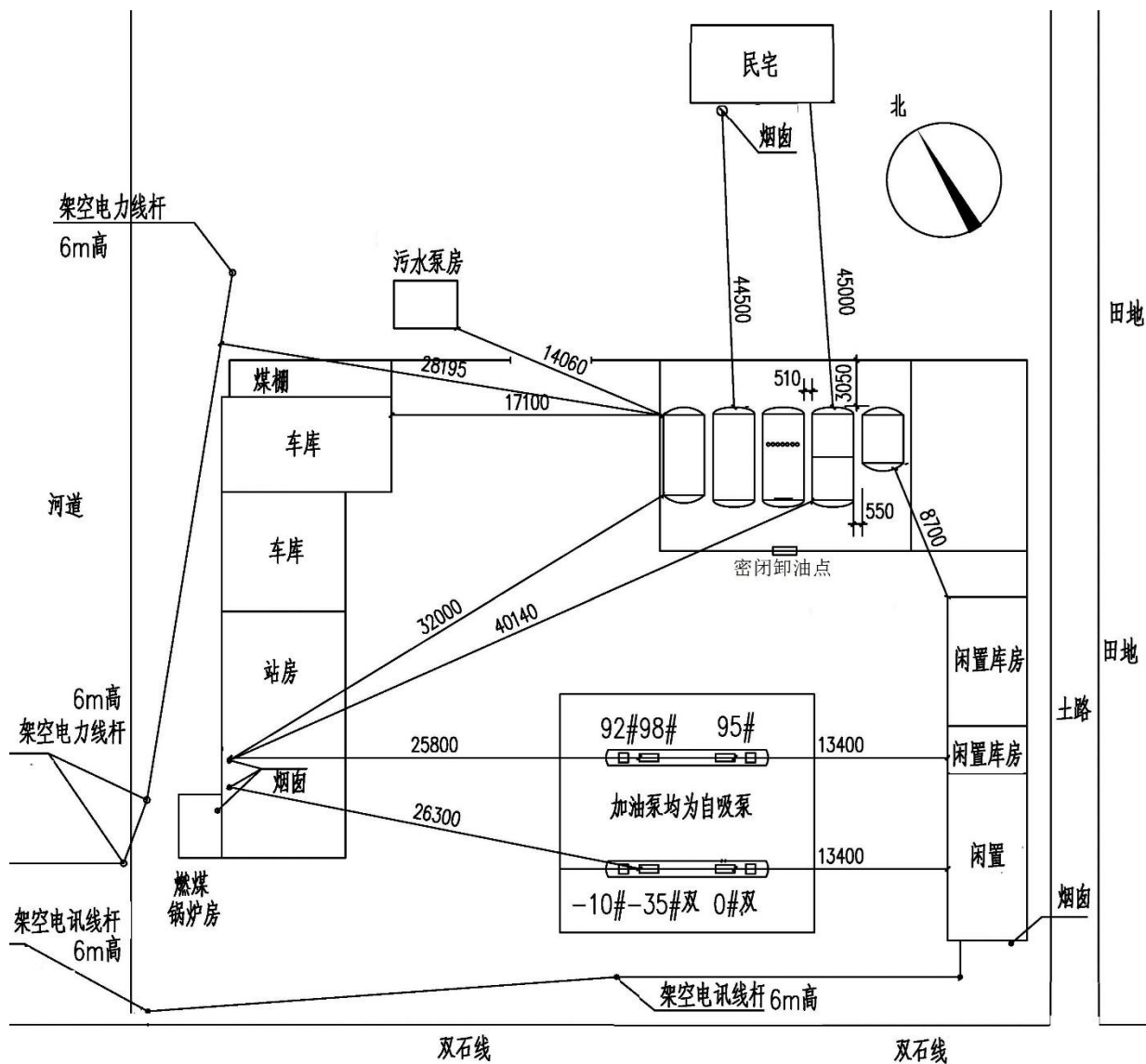
图 2.3-1 周边环境及总平面布置图
