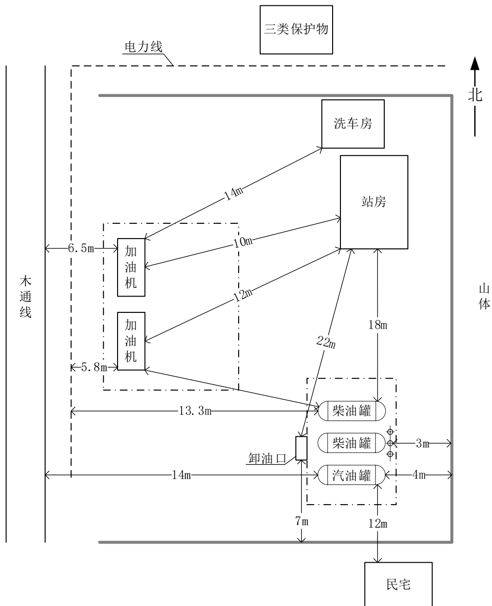
图 2.3-1 加油站周边环境和总平面布置示意图
